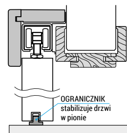
PRZEKRÓJ PIONOWY SYSTEMU PRZESUWNEGO
